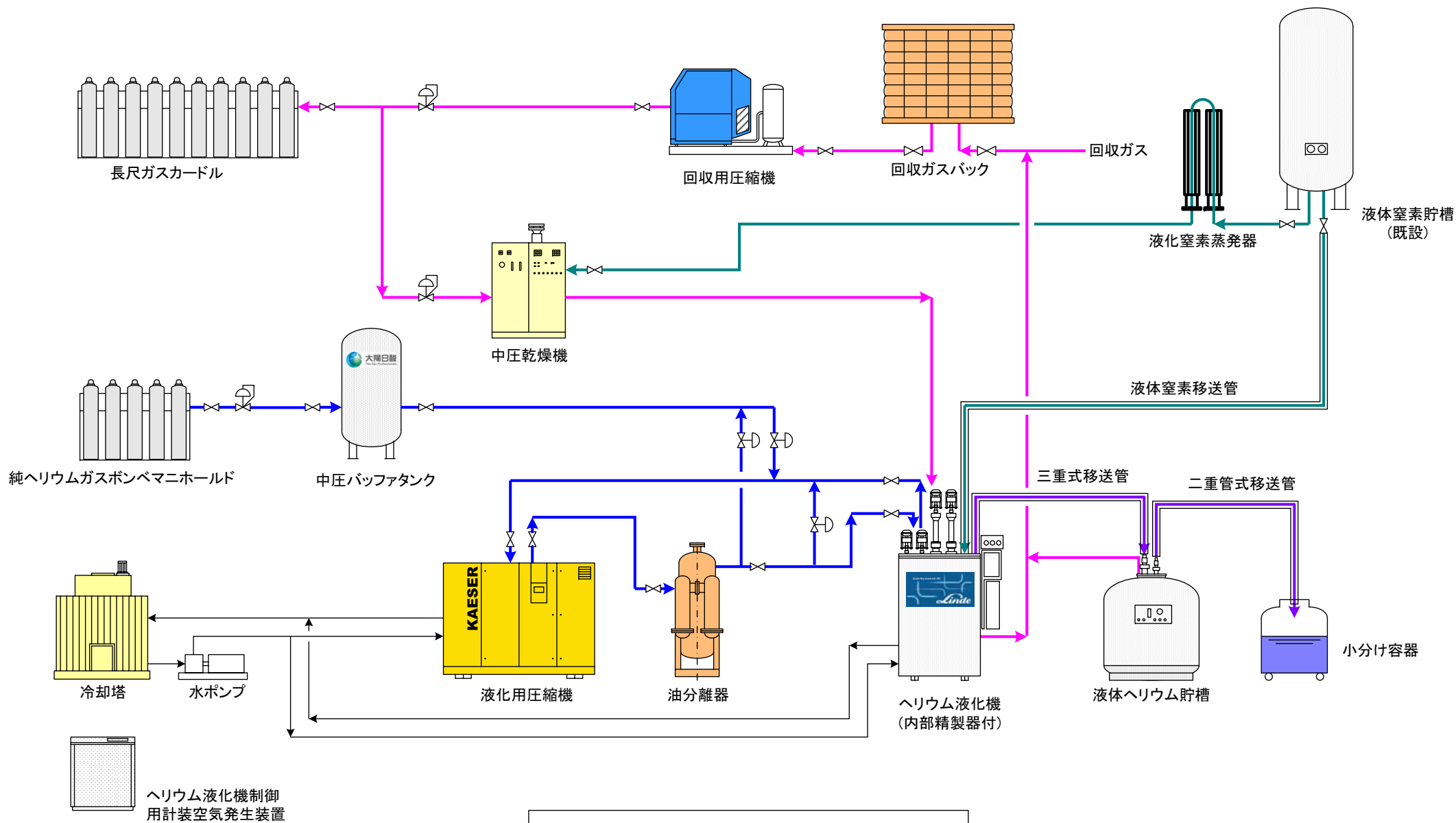
富山大学ヘリウム液化システム機器構成図
